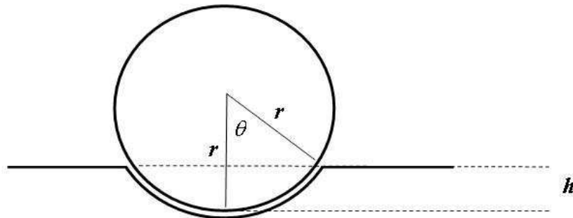
Figura 7.- Si el azote cilíndrico (fusta, caña, etc) se hunde una profundidad h en la piel, la relación entre la profundidad y el ángulo \theta viene dada por la ecuación (9). De (8) puede deducirse la superficie de impacto.
