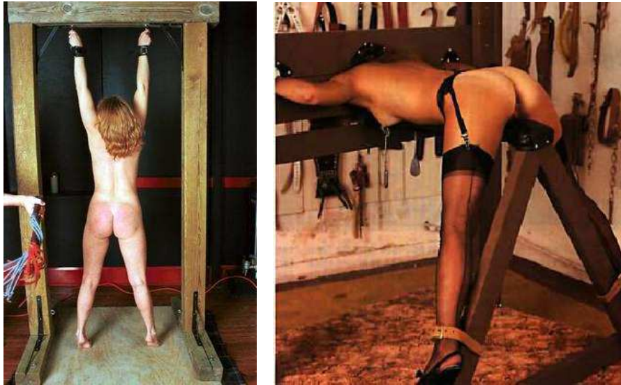
Figura 4.- Izquierda: La suspensión parcial del sujeto (atención: utilizando muñequeras especiales para suspensión) hace que ponga en tensión los músculos de la espalda. Al estar de pie contrae también los bíceps femorales y al estar de puntillas tiene que contraer los gemelos, por lo que los azotes serán más dolorosos en esas zonas. Sin embargo, en esa postura no se contraen las nalgas. En cambio, cuando el sujeto se dobla (derecha), se tensa la zona de las nalgas, al contrario de lo que sucede si el sujeto está estirado boca abajo sobre una superficie plana. Imágenes extraídas de Internet.
